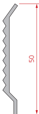
Artikelnummer 151595 (schaal 1:1)
