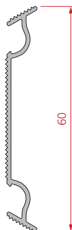
Artikelnummer 151599 (schaal 1:1)
